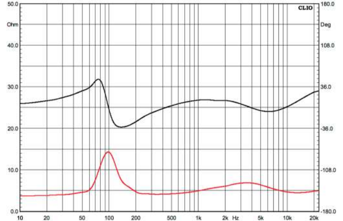
Impedance/Phase
